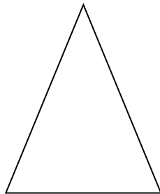
gleichschenkliges Dreieck
