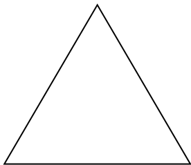
gleichseitiges Dreieck
