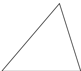
spitzwinkliges Dreieck
