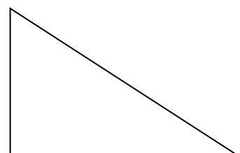
rechtwinkliges Dreieck
