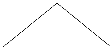
stumpfwinkliges Dreieck
