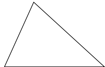
ungleichseitiges Dreieck
